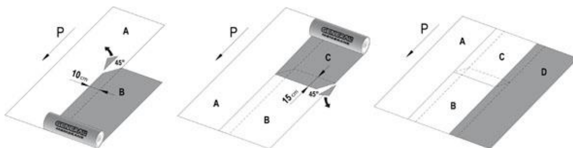
Fig. 9 – posa in MONOSTRATO o PRIMO STRATO: posizionamento teli e esecuzione saldature sezione corrente (le lettere indicano la successione di posa dei foglie con indicazione delle misure delle sovrapposizioni laterali e di testa)
