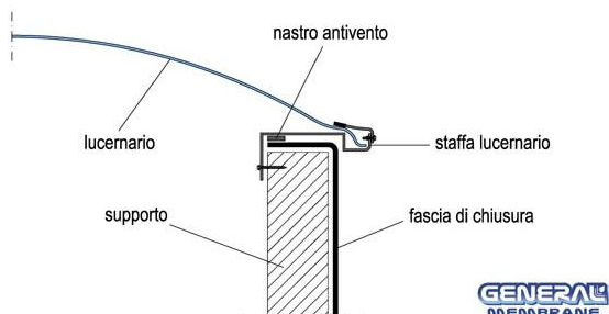
Fig. 28 – risvolto lucernaio in sezione
