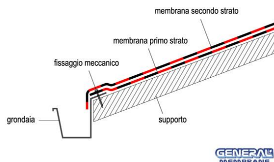
Fig. 35 - Grondaie
