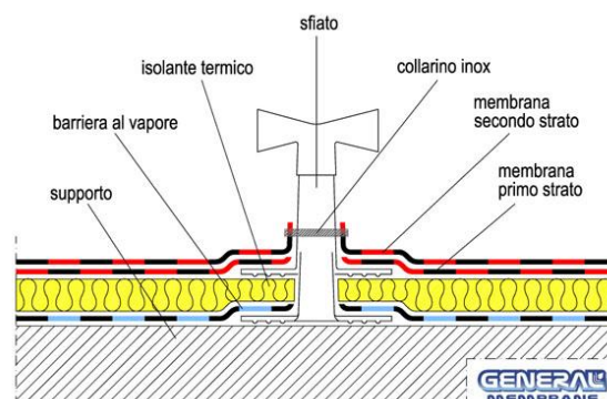
Fig. 23 - Sfiato su estradosso con stratigrafia coibentata
