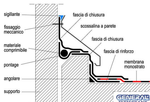
Fig. 33 – Giunto di Dilatazione a Parete
