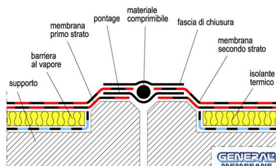
Fig. 31 – Giunto di dilatazione Piatto – tetto caldo
