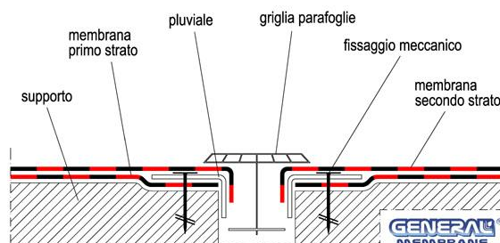
Fig. 14 – Scarico di un Pluviale
