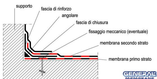
Fig. 19 - risvolto verticale doppio strato – Tipo 3
