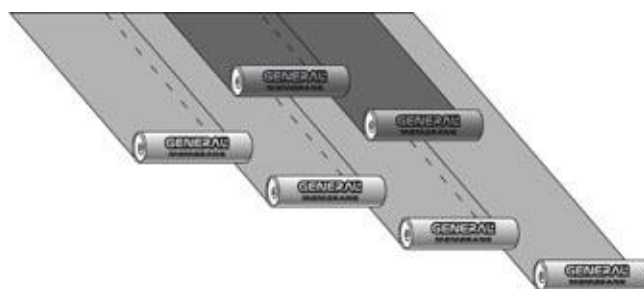
Fig. 8 - Configurazione teli nella posa in doppio strato
