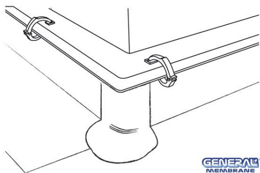
Fig. 29 – lucernaio: rinforzo dell'angolo
