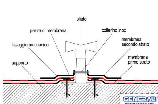
Fig. 22 - Sfiato/Areatore con fissaggio meccanico
