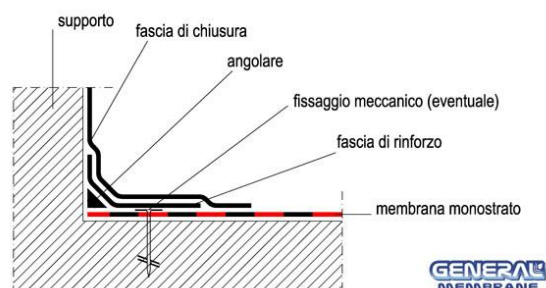
Fig. 16 - risvolto verticale: posa in monostrato con fissaggio meccanico al perimetro
