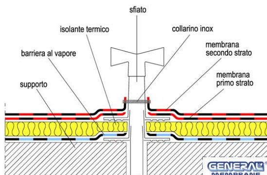
Fig. 24 - Sfiato doppio corpo collegato alla barriera vapore
