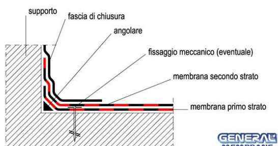
Fig. 18 - risvolto verticale doppio strato – Tipo 2
