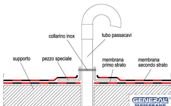
Fig. 26 - Tubo passante con pezzo speciale
