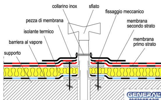
Fig. 25 - Sfiato doppio corpo collegato a ambienti interni
