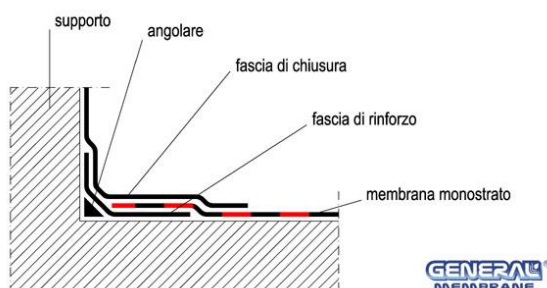
Fig. 15 - risvolto verticale: posa in monostrato senza fissaggio meccanico
