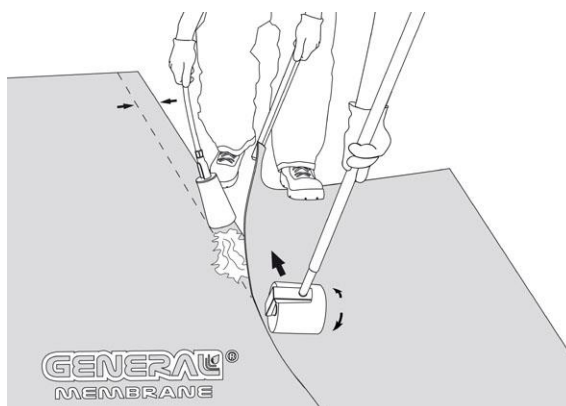
Fig. 5 - Esempio di posa a secco in indipendenza, con sola saldatura delle giunzioni mediante fiamma generata da bruciatore a gas propano
