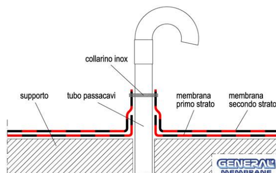
Fig. 27 - Tubo passante senza pezzo speciale
