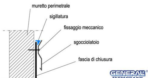
Fig. 20 – coronamento superiore di risvolto verticale: soluzione con profilo metallico a gocciolatoio
