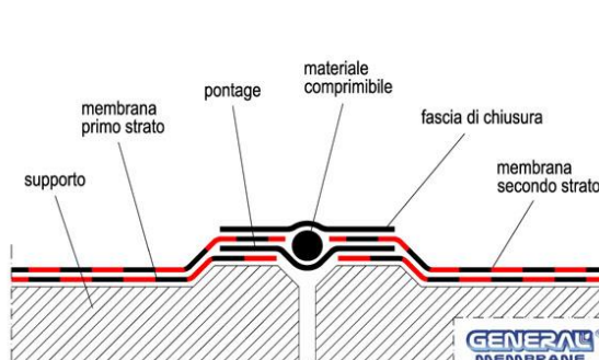
Fig. 30 – Giunto di dilatazione Piatto – tetto freddo
