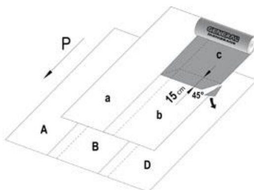
Fig. 10 – posa in DOPPIO STRATO: posizionamento teli e esecuzione saldature sezione corrente (il SECONDO STRATO è indicato con lettere minuscole)
