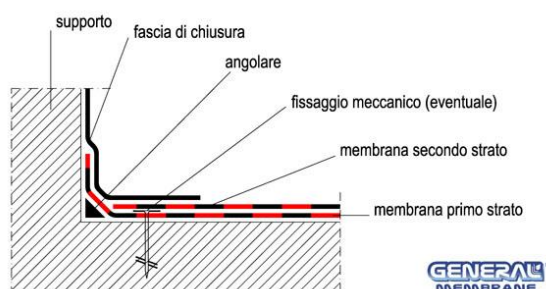
Fig. 17 - risvolto verticale doppio strato – Tipo 1
