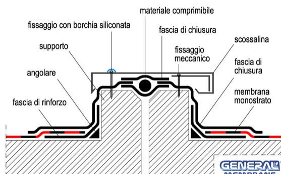
Fig. 32 – Giunto di Dilatazione in Rilievo
