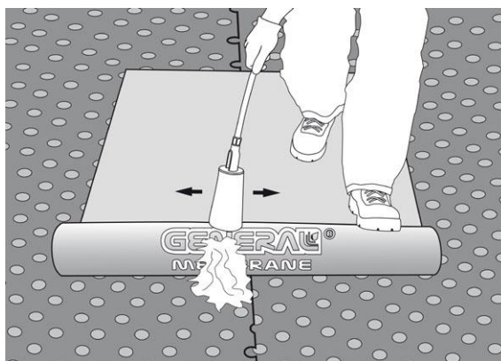
Fig. 4 - Esempio di posa in semiaderenza mediante fiamma generata da bruciatore a gas propano (Membrana forata di base: PEGASUS SPOT non oggetto del presente Certificato)
