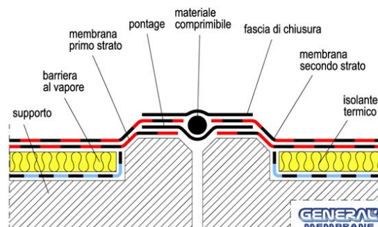
Fig. 32 – Giunto di dilatazione Piatto – tetto caldo
