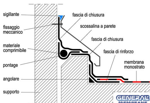
Fig. 34 – Giunto di Dilatazione a Parete
