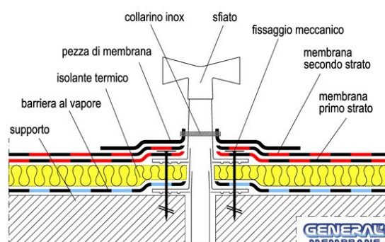
Fig. 26 - Sfiato doppio corpo collegato a ambienti interni
