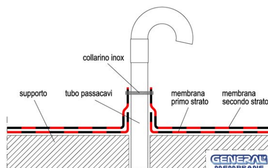
Fig. 28 - Tubo passante senza pezzo speciale
