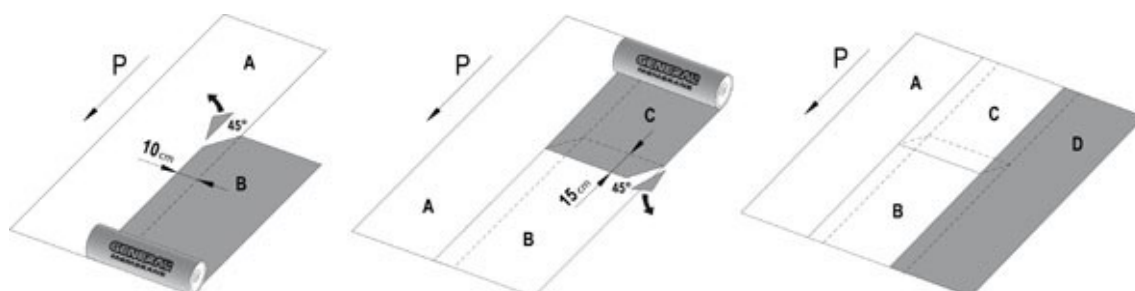
Fig. 10 – posa in MONOSTRATO o PRIMO STRATO: posizionamento teli e esecuzione saldature sezione corrente (le lettere indicano la successione di posa dei fogli con indicazione delle misure delle sovrapposizioni laterali e di testa)
