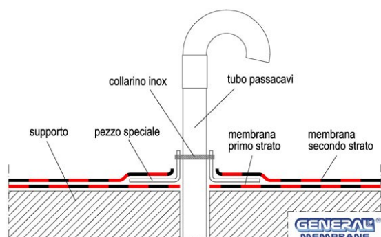
Fig. 27 - Tubo passante con pezzo speciale
