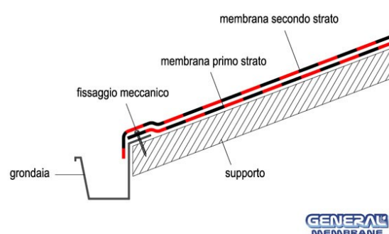
Fig. 36 - Grondaie
