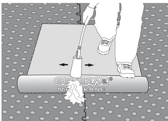
Fig. 5 - Esempio di posa in semiaderenza mediante fiamma generata da bruciatore a gas propano (Membrana forata di base: PEGASUS SPOT non oggetto del presente Certificato)
