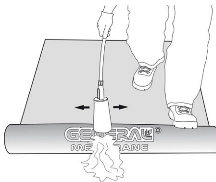
Fig. 2 - Esempio di posa in totale aderenza mediante fiamma generata da bruciatore a gas propano
