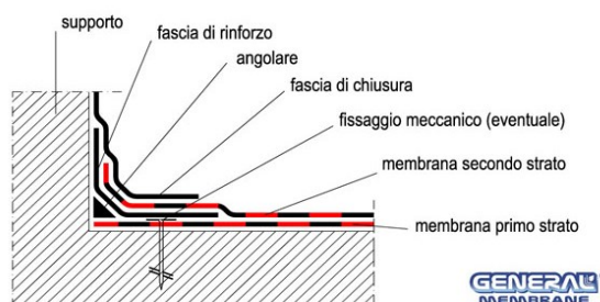
Fig. 20 - risvolto verticale doppio strato – Tipo 3
