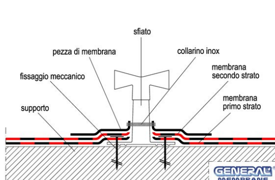
Fig. 23 - Sfiato/Areatore con fissaggio meccanico
