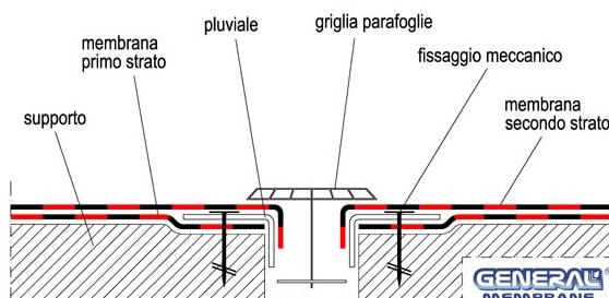
Fig. 15 – Scarico di un Pluviale
