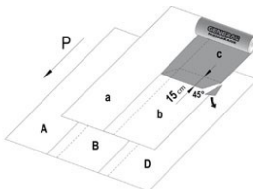
Fig. 11 – posa in DOPPIO STRATO: posizionamento teli e esecuzione saldature sezione corrente (il SECONDO STRATO è indicato con lettere minuscole)
