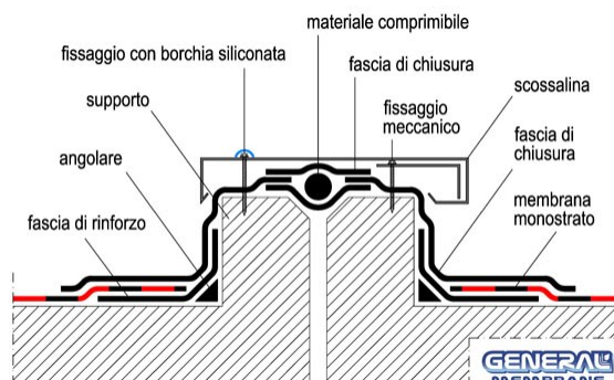
Fig. 33 – Giunto di Dilatazione in Rilievo
