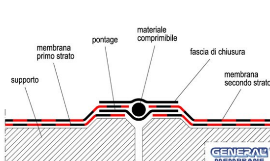
Fig. 31 – Giunto di dilatazione Piatto – tetto freddo
