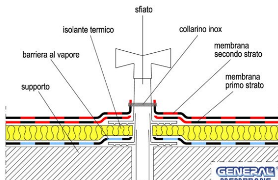
Fig. 25 - Sfiato doppio corpo collegato alla barriera vapore
