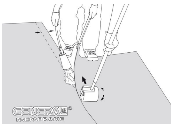
Fig 6 - Esempio di posa a secco in indipendenza, con sola saldatura delle giunzioni mediante fiamma generata da bruciatore a gas propano
