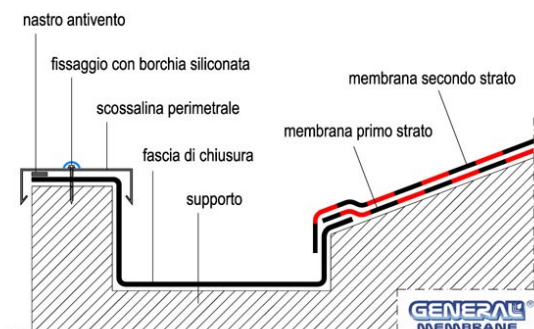
Fig. 35 - Canali di Gronda
