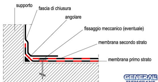
Fig. 18 - risvolto verticale doppio strato – Tipo 1
