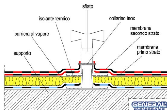
Fig. 24 - Sfiato su estradosso con stratigrafia coibentata
