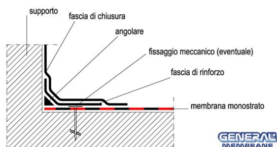
Fig. 17 - risvolto verticale: posa in monostrato con fissaggio meccanico al perimetro
