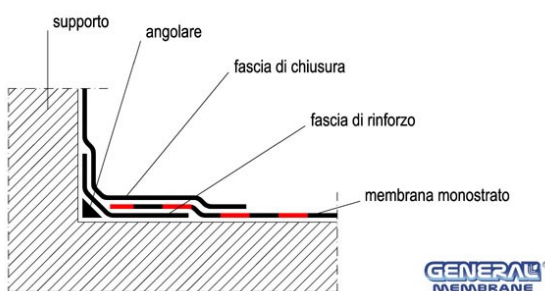
Fig. 16 - risvolto verticale: posa in monostrato senza fissaggio meccanico
