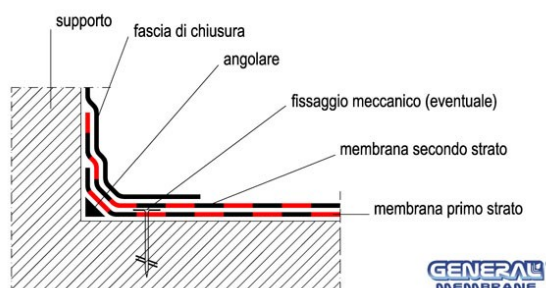
Fig. 19 - risvolto verticale doppio strato – Tipo 2
