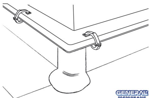
Fig. 30 – lucernaio: rinforzo dell’angolo
