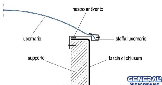
Fig. 29 – risvolto lucernaio in sezione
